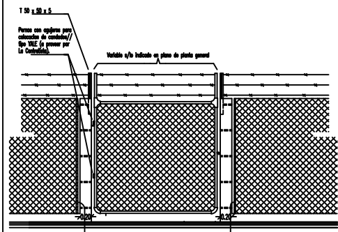
TRAMO DESMONTABLE En caso de posibilidad de salida de agua en hora puntual de lavados dentro el cerco.
