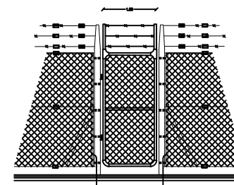
PUERTA SIMPLE
