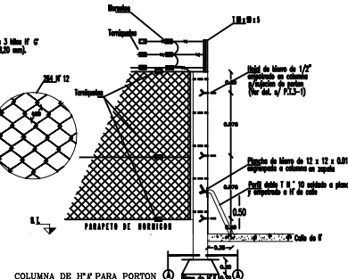
COLUMNA DE H/F PARA PORTON
