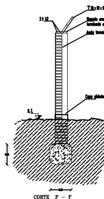
CORTE F - F
