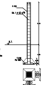
DETALLE ESTRUCTURA
