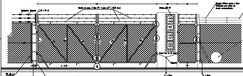
DETALLE PORTON DE INGRESO
