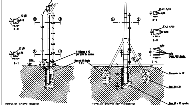
DETALLE POSTE SIMPLE
