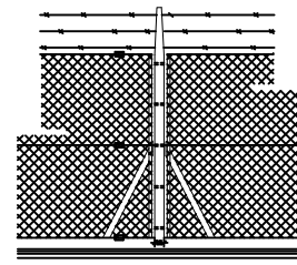
POSTE DE REFUERZO (solo 15.00 mts.)
