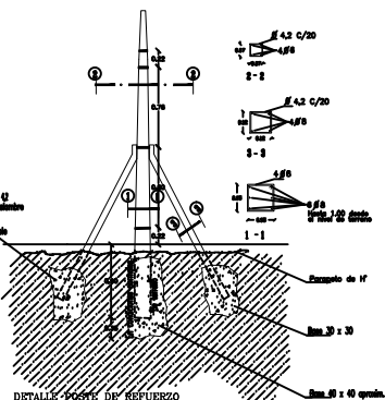
DETALLE POSTE DE REFUERZO
