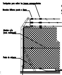
POSTE ESQUINERO
