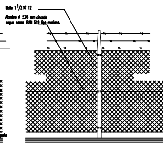
POSTE SIMPLE (solo 3.00 mts.)
