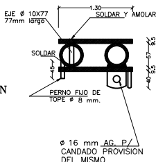
CORTE B-B
