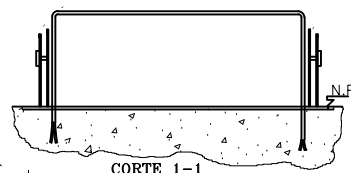
CORTE 1-1
