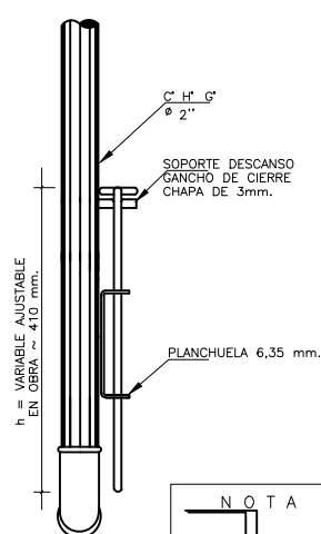
CORTE B-B
