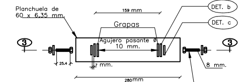
DETALLE 4 TOPE DE FIJACION DE PORTON
