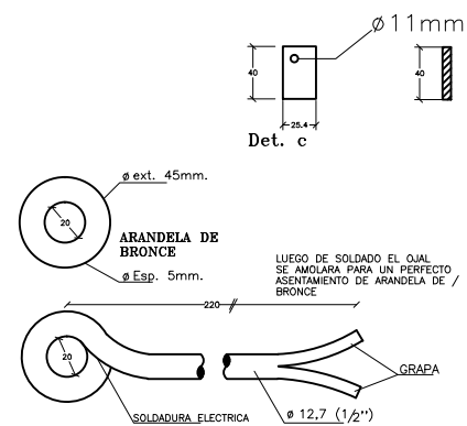
DETALLE 4 TOPE DE FIJACION DE PORTON
