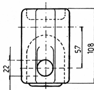
AISLADOR ROLDANA MN 16 (ANSI 53-1)
