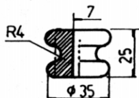
AISLADOR ROLDANA MN 15
