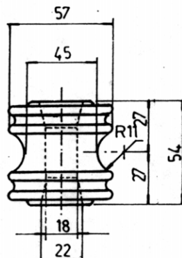
AISLADOR ROLDANA MN 16 (ANSI 53-1)
