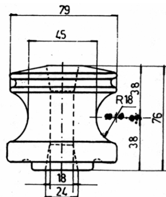
AISLADOR ROLDANA MN 17 (ANSI 53-2)
