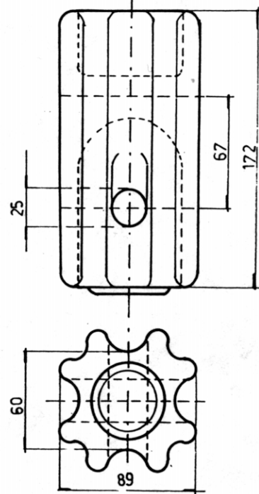
AISLADOR PARA RIENDA MN 21 (ANSI 54-4)
