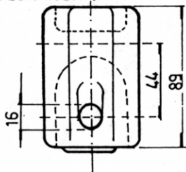
AISLADOR PARA RIENDA MN 20 (ANSI 54-1)
