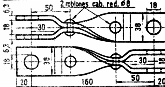
PIEZA INTERMEDIA HH A 90° Q113
