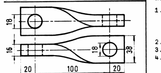
OREJA DOBLE A 90° Q125
