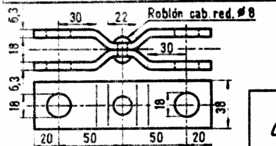
PIEZA INTERMEDIA HH Q115
