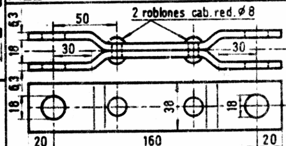
PIEZA INTERMEDIA HH LARGA Q114
