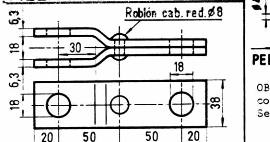
PIEZA INTERMEDIA MH Q116
