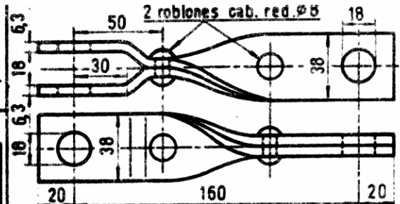
PIEZA INTERMEDIA MH A 90° Q110
