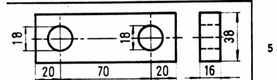
OREJA DOBLE PLANA Q126
